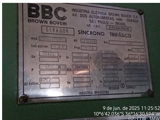
Nameplate data: Alternator/ Generator nº 2 (UTE Coruripe Usina COR)
